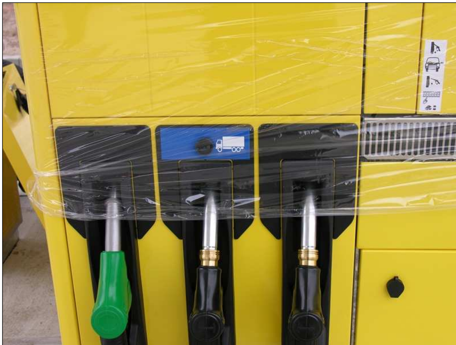
Montaż odmierzaczy na stacji paliw typ: Quantum 500T1 HS 3-6
